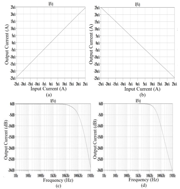
Figure 4. DC Analysis for Input Stage: (a) I_z=I_p-I_n ( I_p variable, I_n=0 ) (b) I_z=I_p-I_n ( I_n variable, I_p=0 ) AC Analysis for Input Stage: (c) I_z=I_p-I_n ( I_p variable, I_n=0 ) (d) I_z=I_p-I_n ( I_n variable, I_p=0 )
